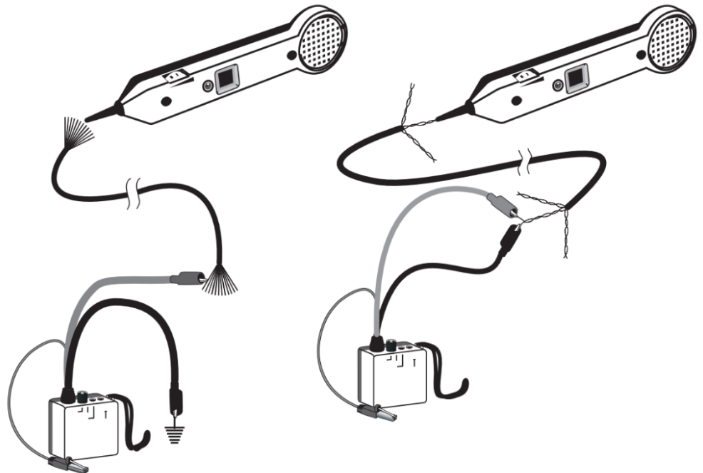
Рисунок 5 – Отбор кабельных пар на удаленном конце кабеля
