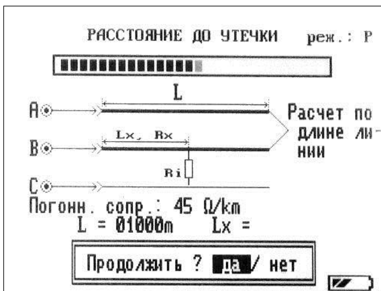
Рисунок 6-18 Метод Муррея
