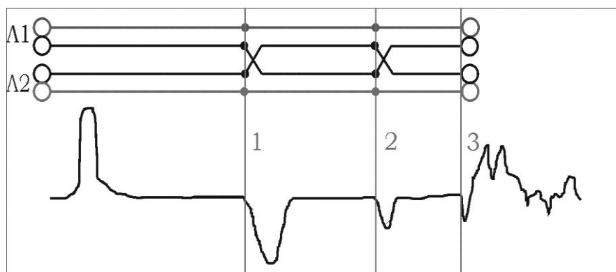
Рисунок 6-8 «Разбитость пар»
