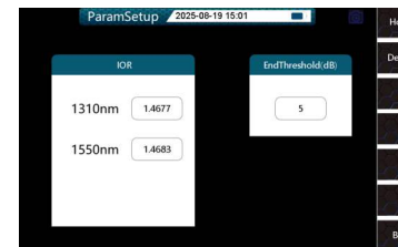
ParamSetup
