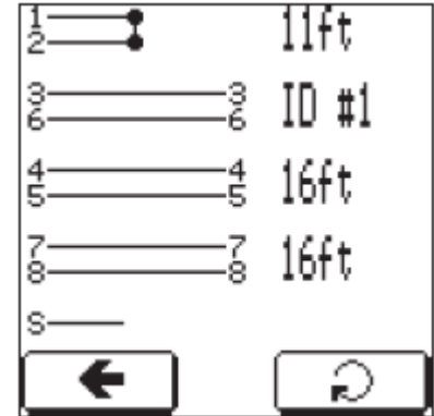
Разводка проводов с коротким замыканием на расстоянии 11 футов на паре 1-2 и отсоединенным экраном.
