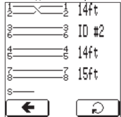
Разводка проводов с обратным подключением пары 1-2 и отсоединенным экраном.
