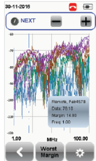
Перекрестные помехи на ближнем конце
