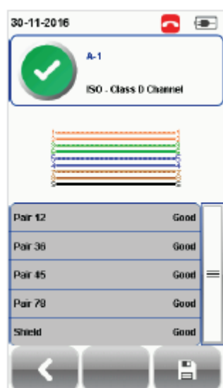
Разводка проводов
