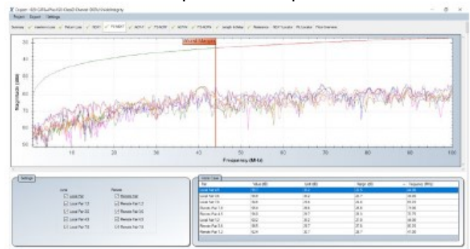
PS-NEXT
