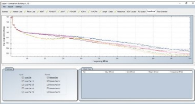
Импеданс
