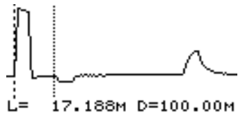
Ответвление с КЗ на конце
