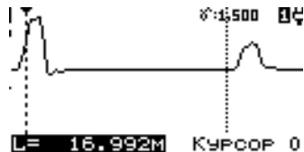
Неправильная установка Рисунок 53
