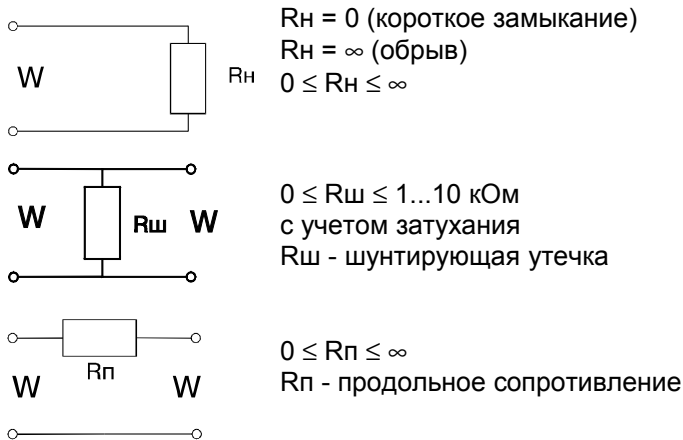
Рисунок 3 - Эквивалентные схемы повреждений
