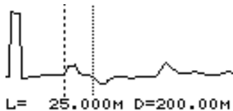
Ответвление от линии
