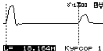
Правильная установка Рисунок 54
