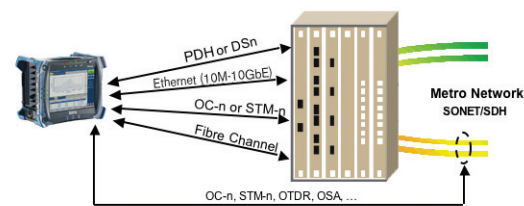
С помощью этой модульной, мультислотовой конструкции платформы FTB-500, пользователи могут настраивать и модернизировать свои системы, согласно выполняемым тестам, и минимизировать капитальные вложения в оборудование.
