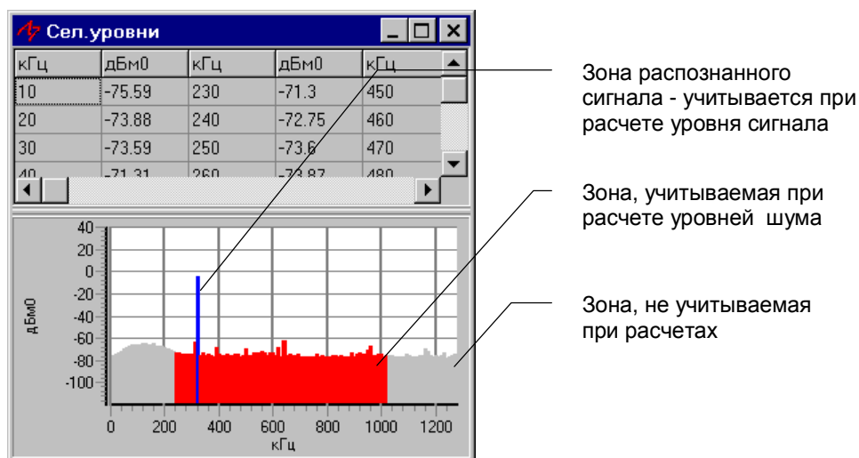
Рис. 36 Селективные уровни
