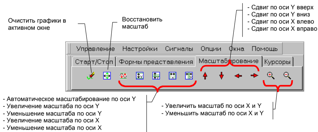
Рис. 28 Масштабирование графиков
