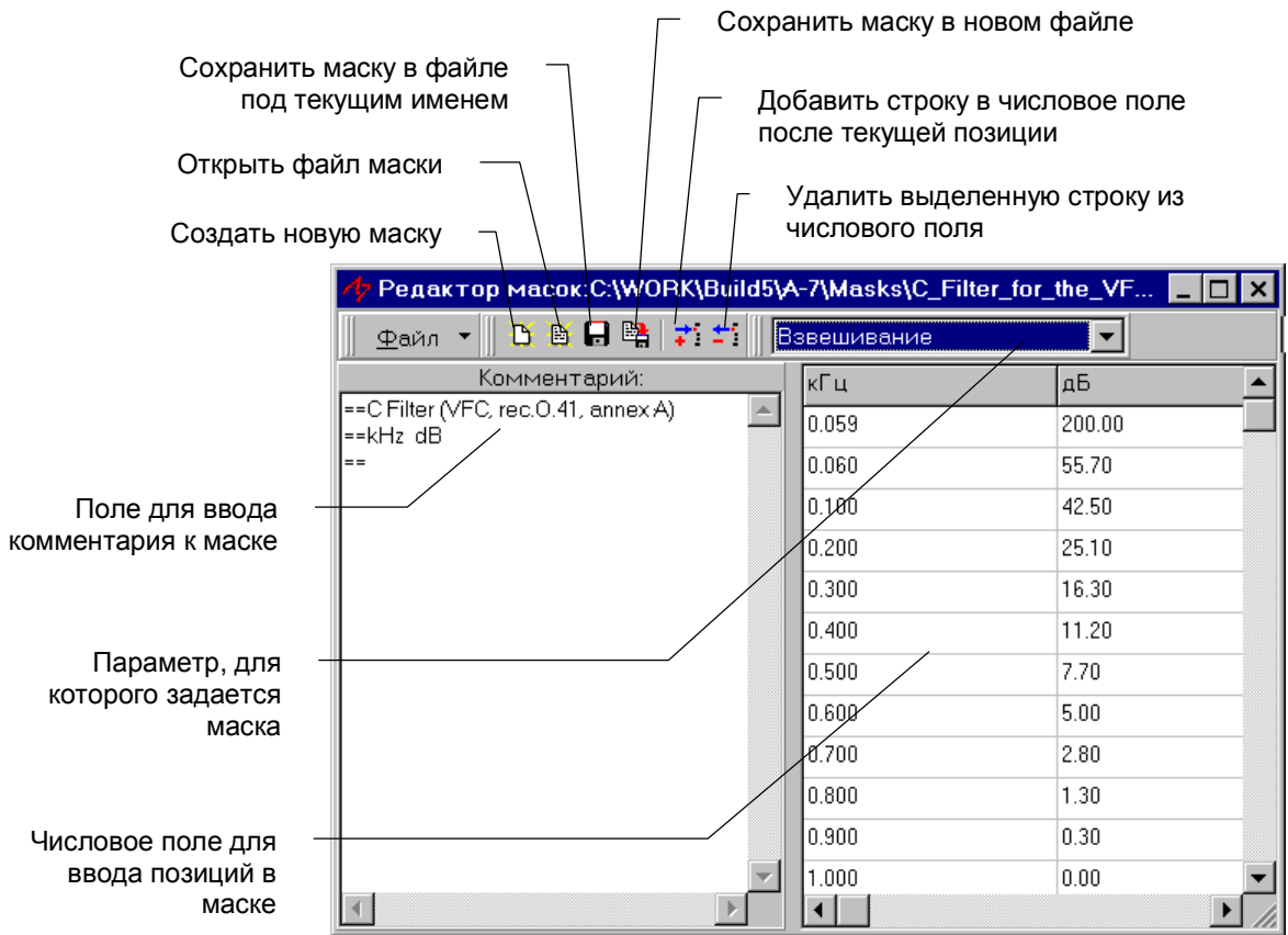
Рис. 16 Редактор масок
