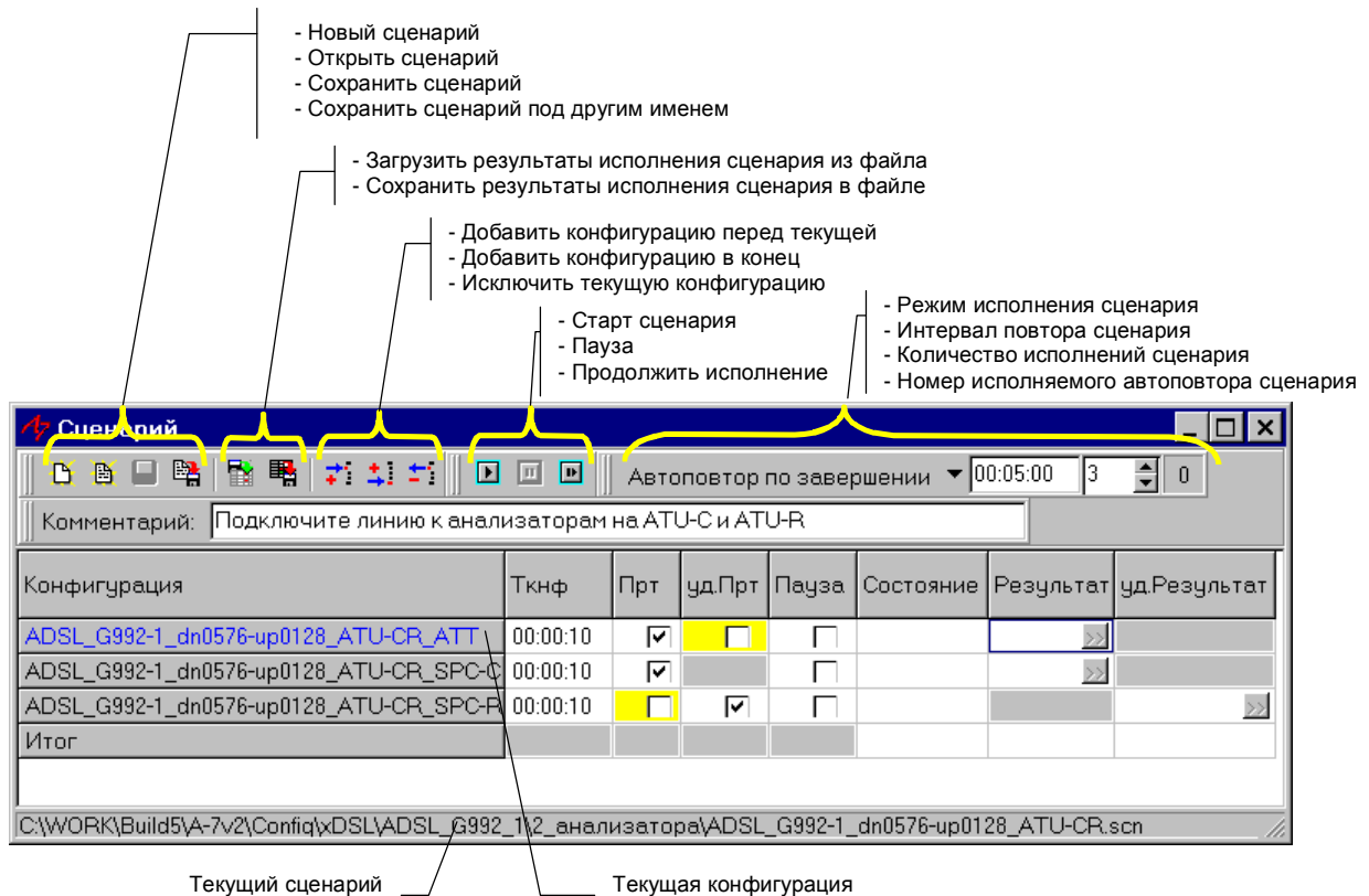
Рис. 20 Форма "Сценарий"
