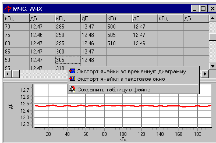
Рис. 27 Таблица характеристики
