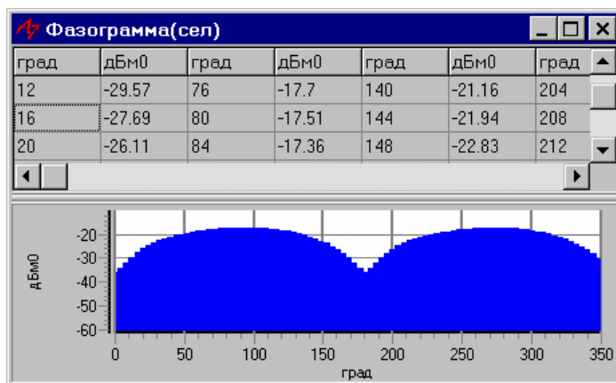
Рис. 38 Форма "Фазограмма(сел)"
