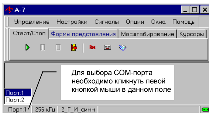
Рис. 2 Выбор COM-порта.
