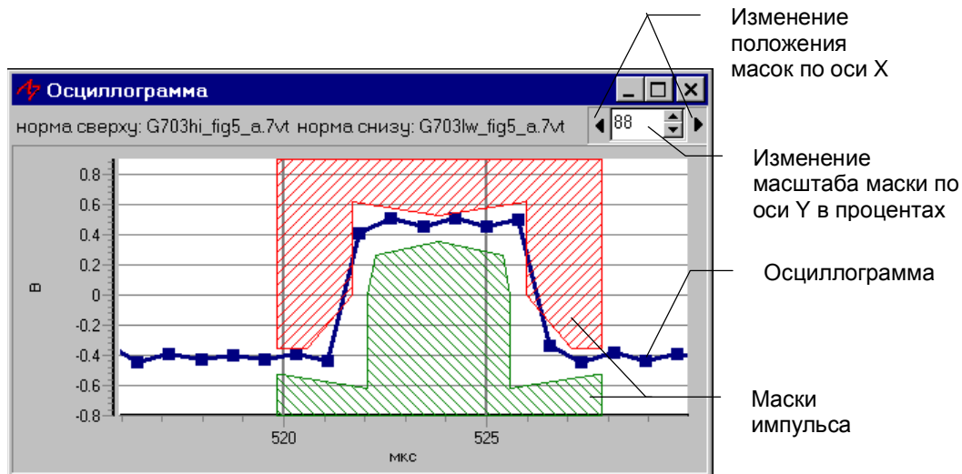
Рис. 35 Маски импульса
